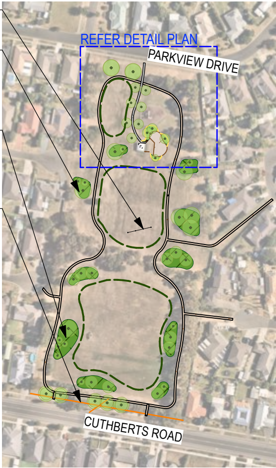
1 SITE PLAN Scale: 1:3000
